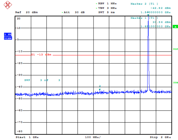
Band25-1.4MHz-QPSK-26047-1RB#0-Range2:1000~2000MHz
