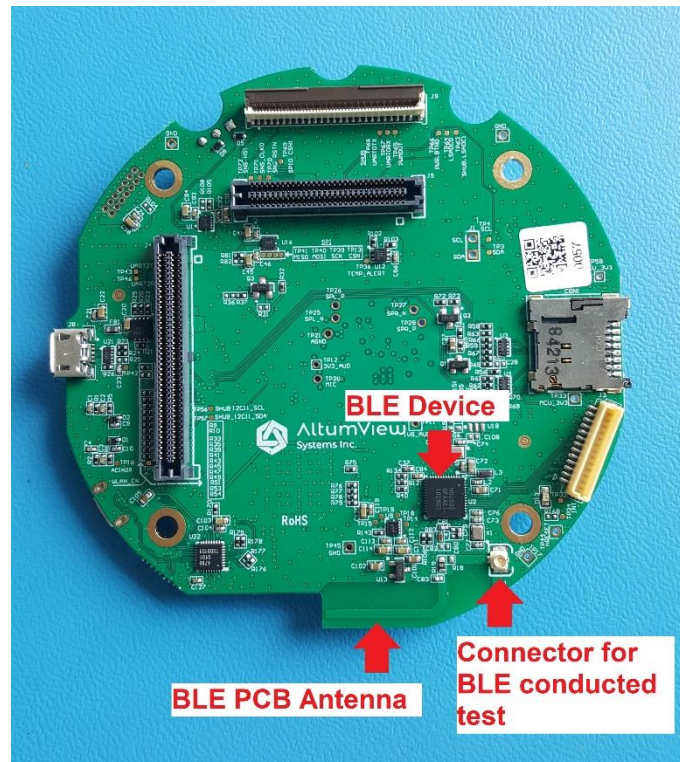
Figure 17 - BLE antenna
