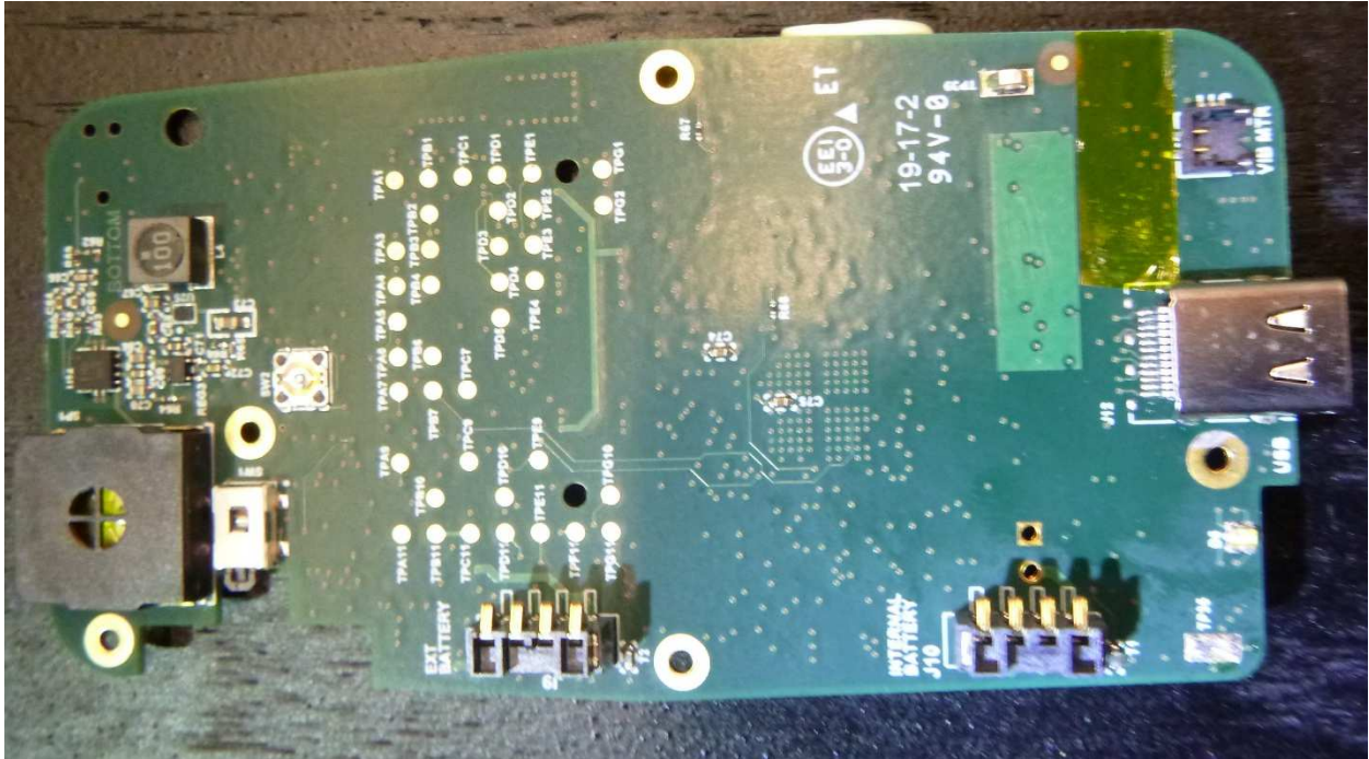
PCB Bottom
