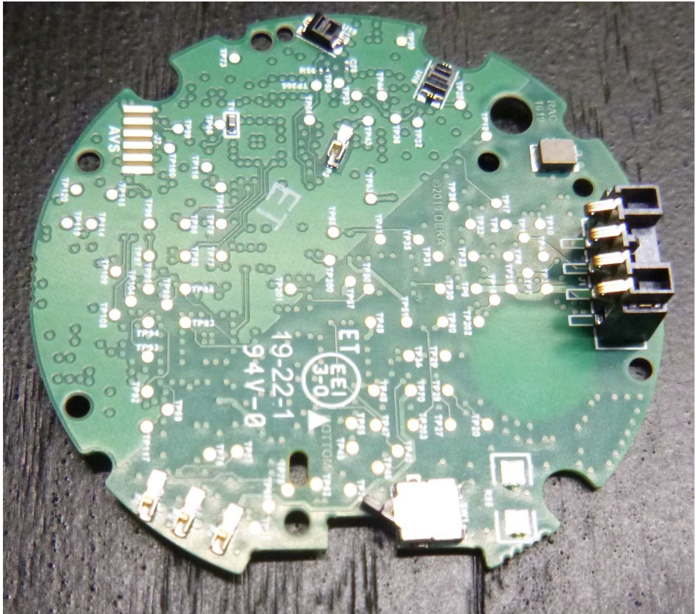
PCB Top
