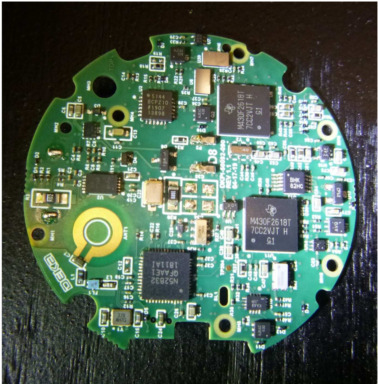
PCB Bottom
