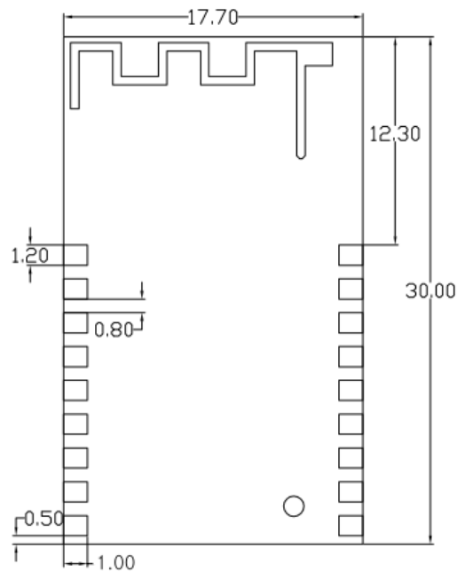
Fig 3 BL3372-P Module Dimensions
