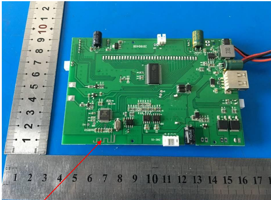
BT ANT
