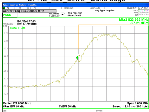
EGPRS 850 Lower Band edge
