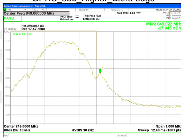
EGPRS 850 Higher Band edge
