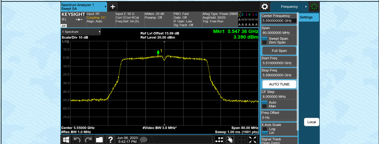
11N40MIMO-Ant1-5550
