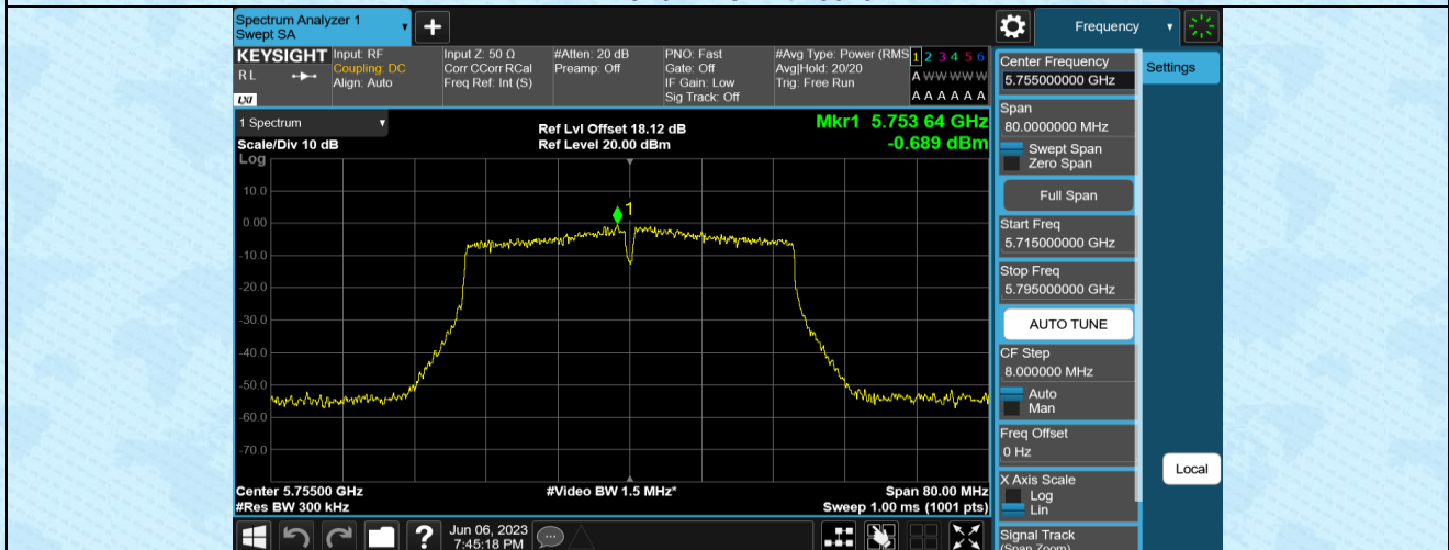
11AC40MIMO-Ant1-5755
