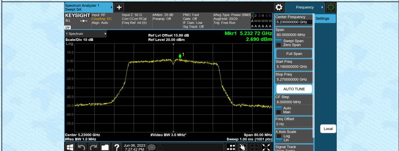
11AC40MIMO-Ant1-5230
