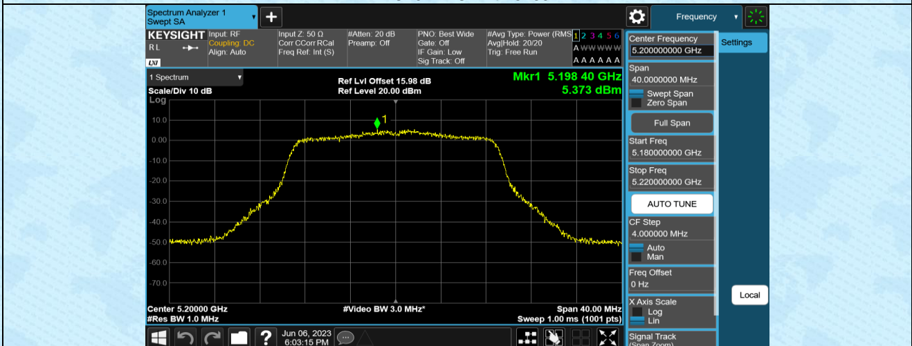
11AC20MIMO-Ant1-5200
