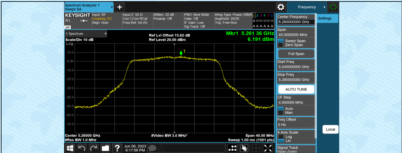
11AC20MIMO-Ant1-5260
