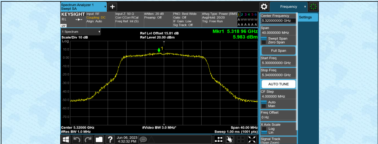
11N20MIMO-Ant1-5320
