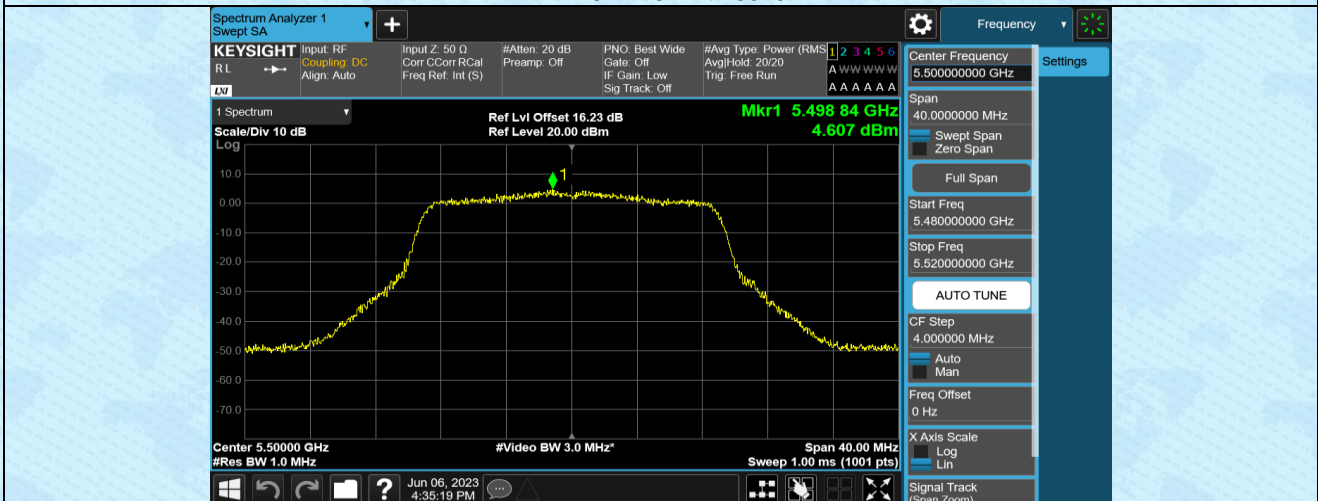
11N20MIMO-Ant1-5500
