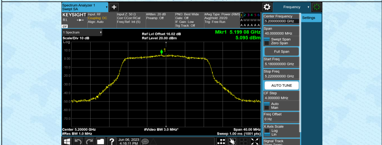
11N20MIMO-Ant1-5200
