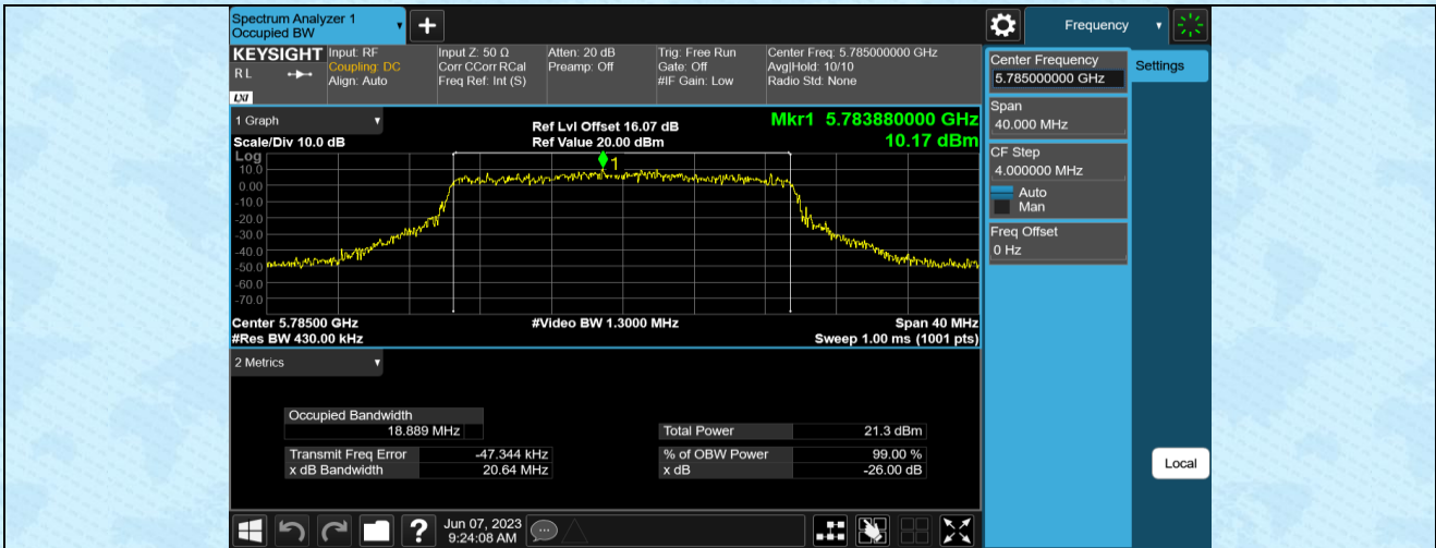
11AX20MIMO-Ant1-5785
