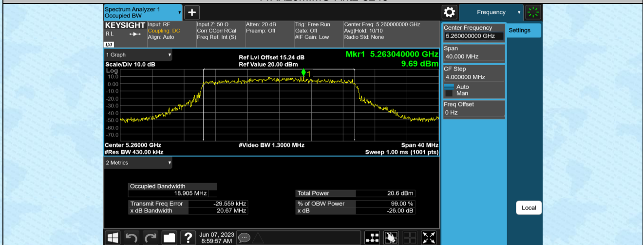
11AX20MIMO-Ant1-5260
