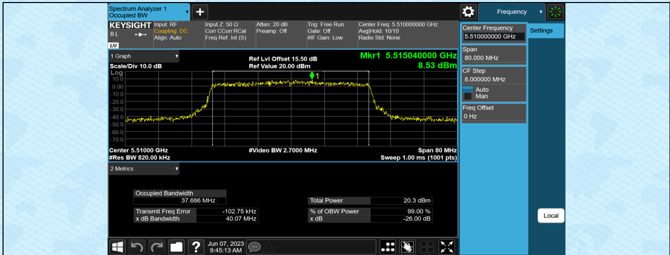
11AX40MIMO-Ant1-5510
