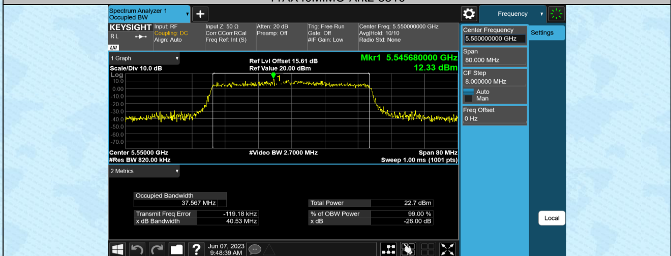
11AX40MIMO-Ant1-5550
