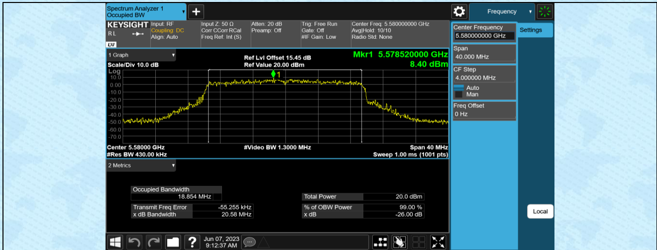
11AX20MIMO-Ant1-5580
