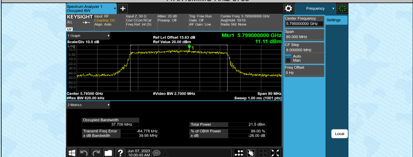
11AX40MIMO-Ant1-5795
