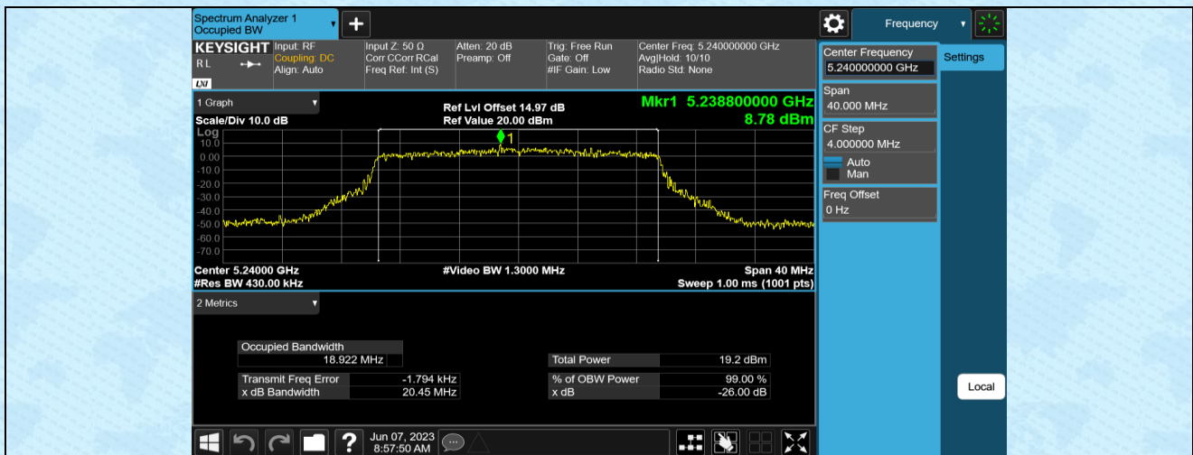
11AX20MIMO-Ant2-5240
