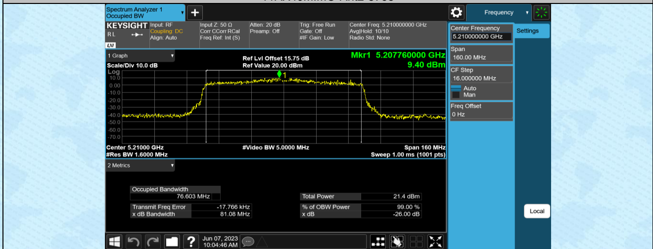
11AX80MIMO-Ant1-5210
