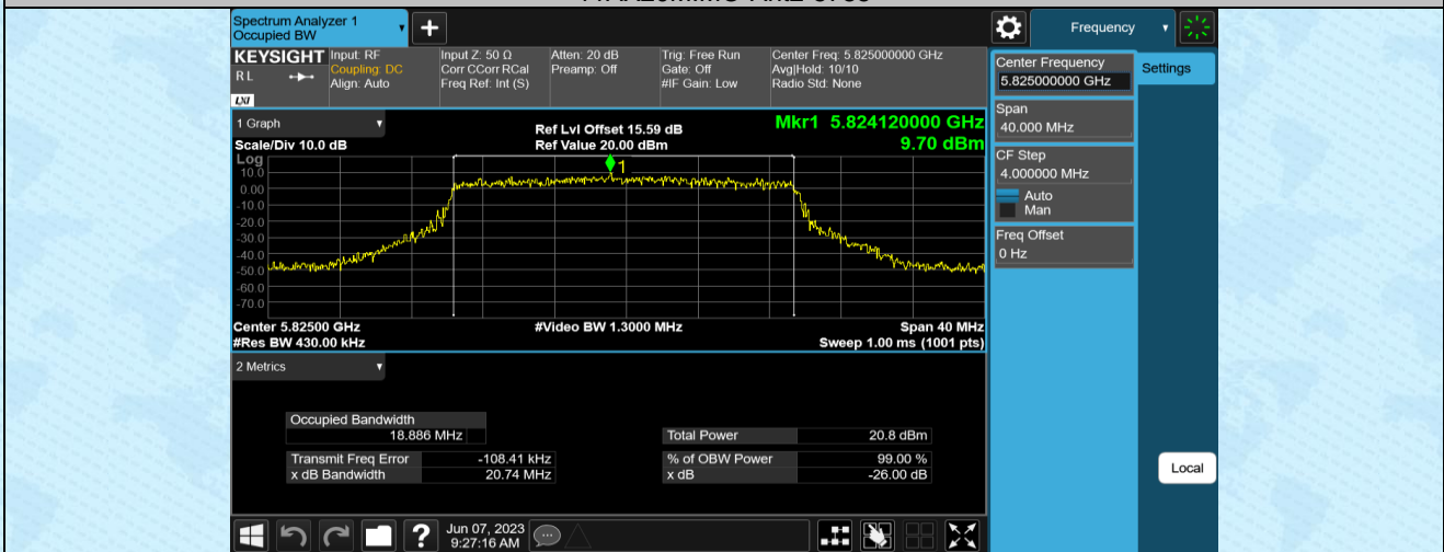
11AX20MIMO-Ant1-5825
