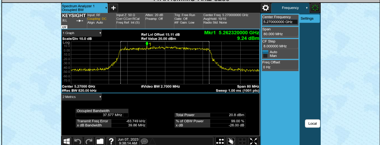
11AX40MIMO-Ant1-5270
