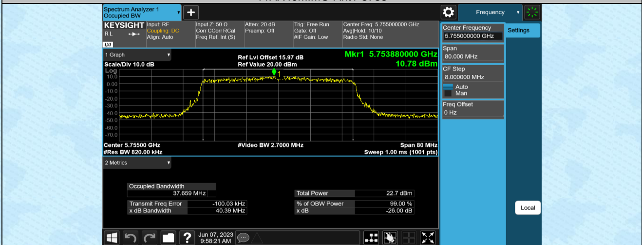
11AX40MIMO-Ant2-5755
