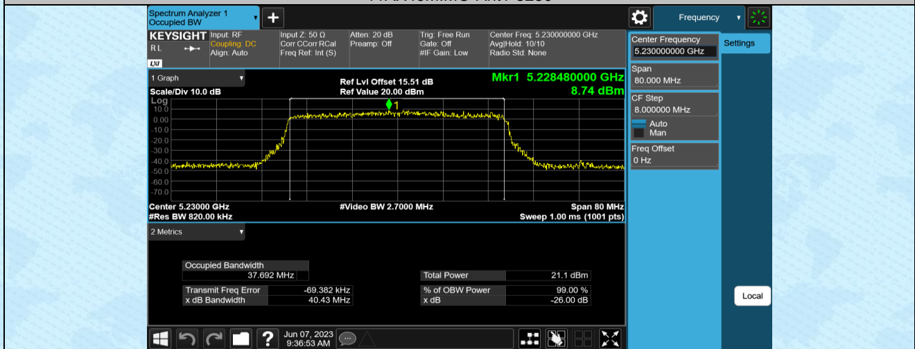
11AX40MIMO-Ant2-5230
