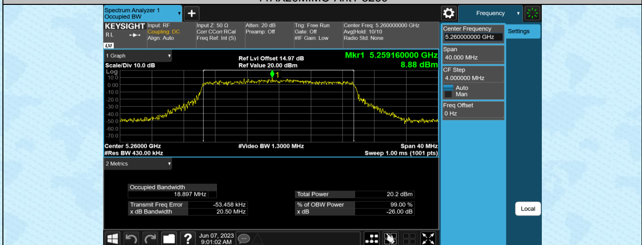
11AX20MIMO-Ant2-5260
