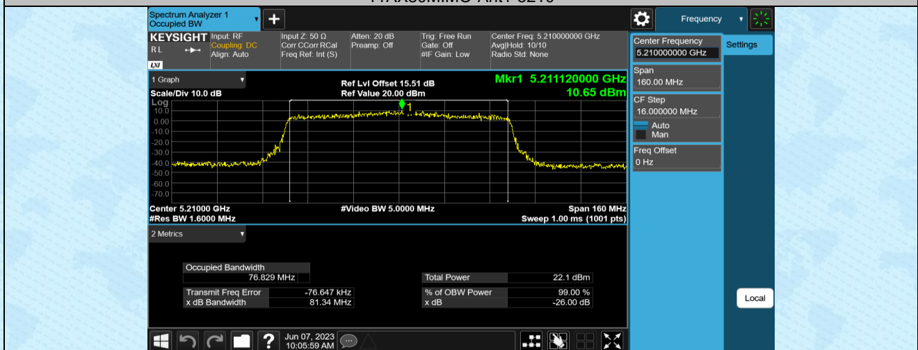
11AX80MIMO-Ant2-5210
