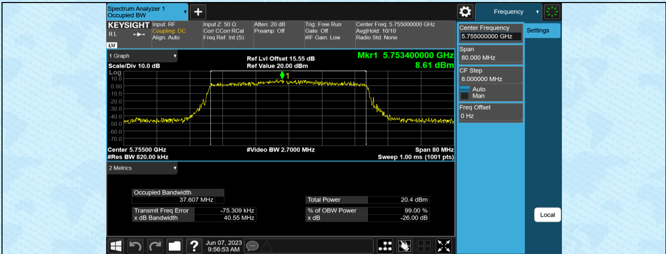
11AX40MIMO-Ant1-5755
