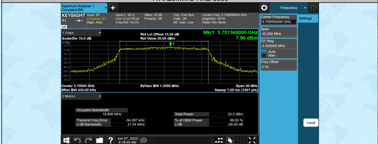
11AX20MIMO-Ant1-5700
