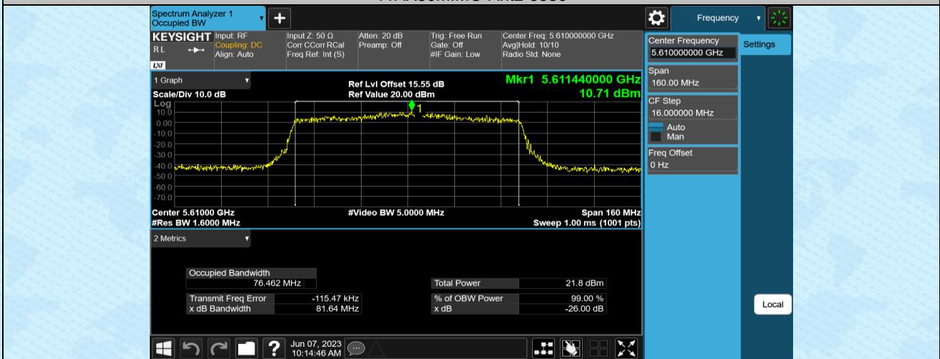
11AX80MIMO-Ant1-5610
