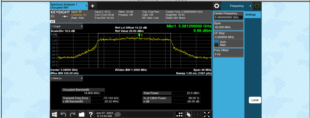
11AX20MIMO-Ant2-5580
