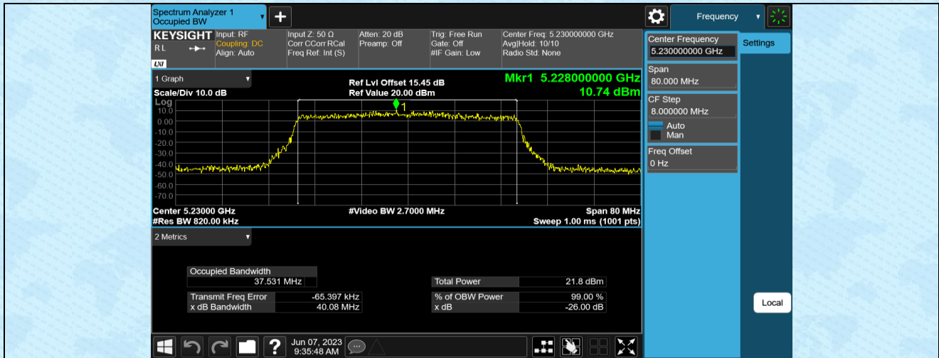
11AX40MIMO-Ant1-5230
