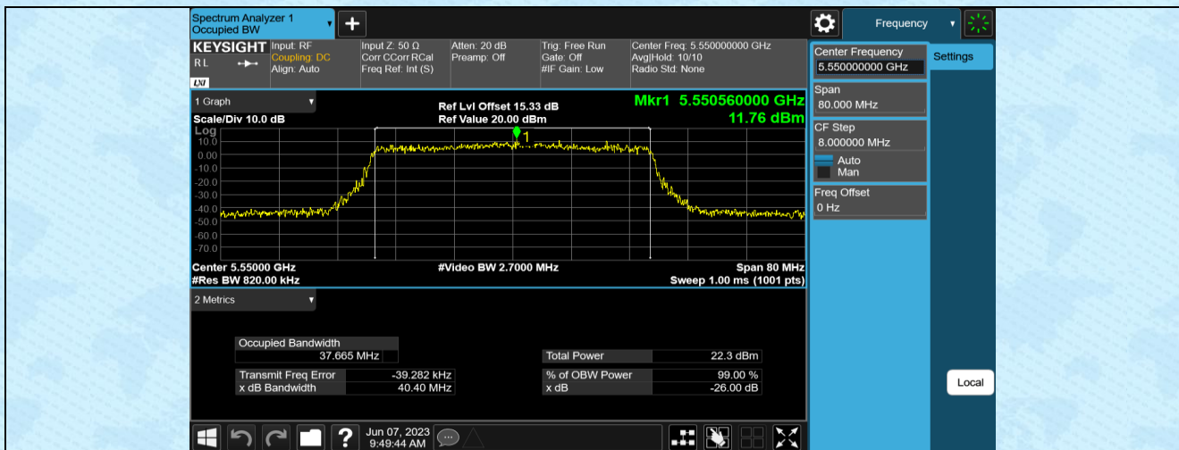
11AX40MIMO-Ant2-5550
