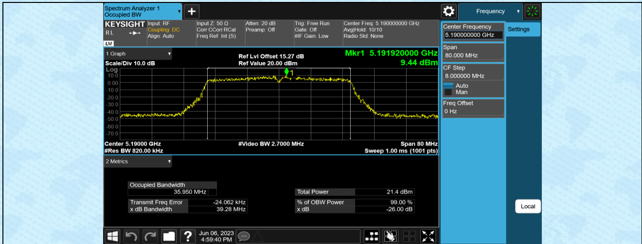
11N40MIMO-Ant1-5190
