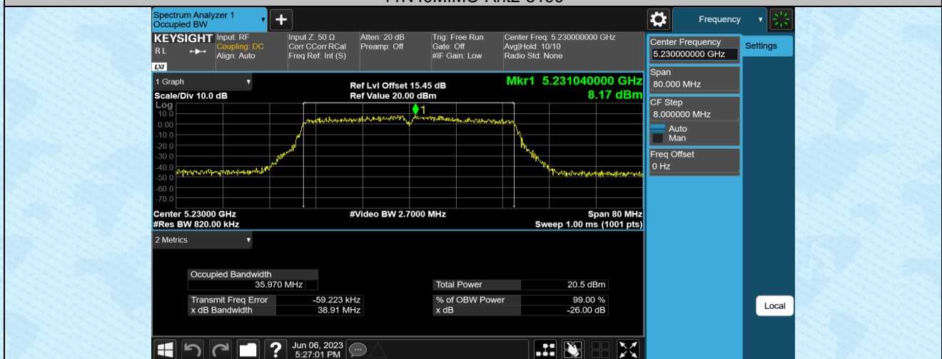
11N40MIMO-Ant1-5230
