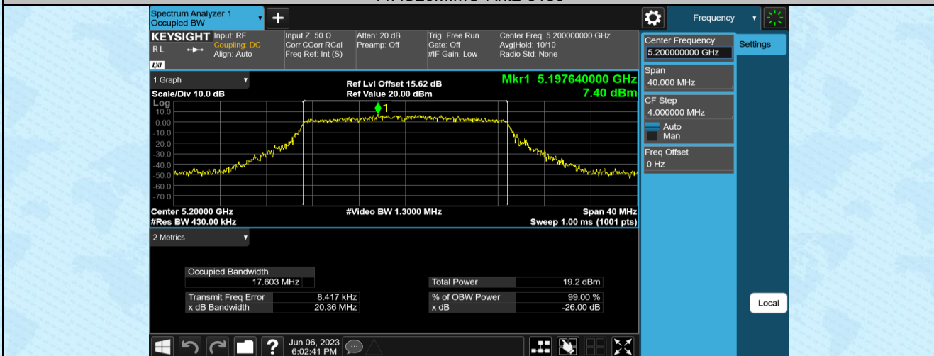
11AC20MIMO-Ant1-5200
