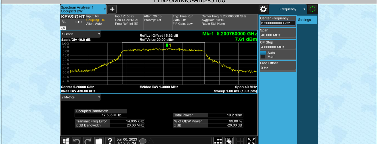
11N20MIMO-Ant1-5200
