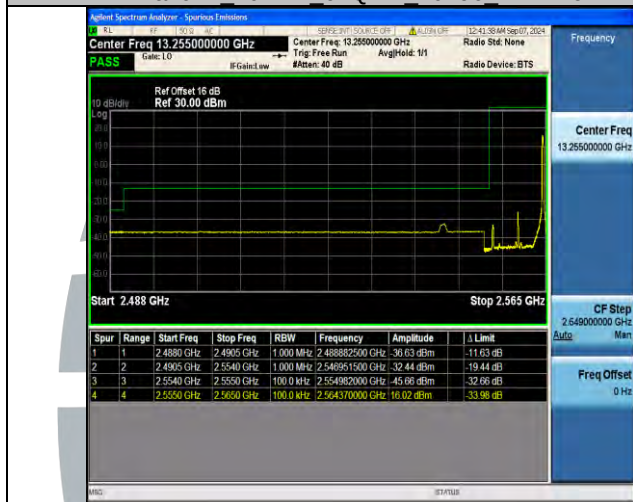
Band41 10MHz 64QAM 41190 1RB#0
