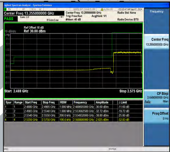
Band41 20MHz QPSK 41140 1RB#99
