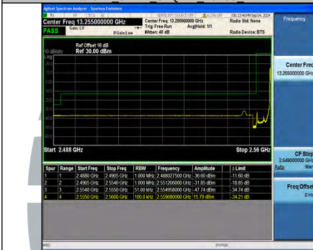
Band41 5MHz 64QAM 40265 1RB#24
