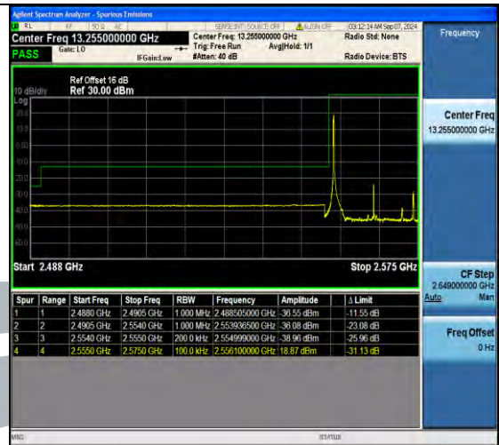
Band41 20MHz QPSK 40340 100RB#0
