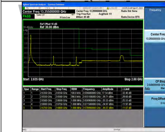
Band41 20MHz QPSK 41140 100RB#0
