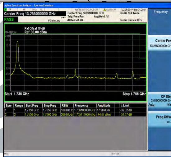
Band4 20MHz 64QAM 20300 100RB#0
