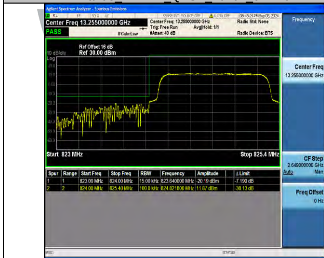
Band5 1.4MHz QPSK 20643 1RB#5
