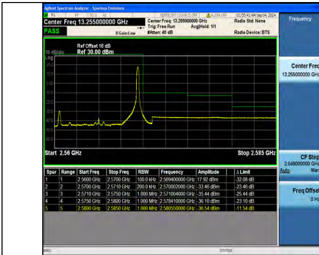
Band7 10MHz 16QAM 20800 1RB#0
