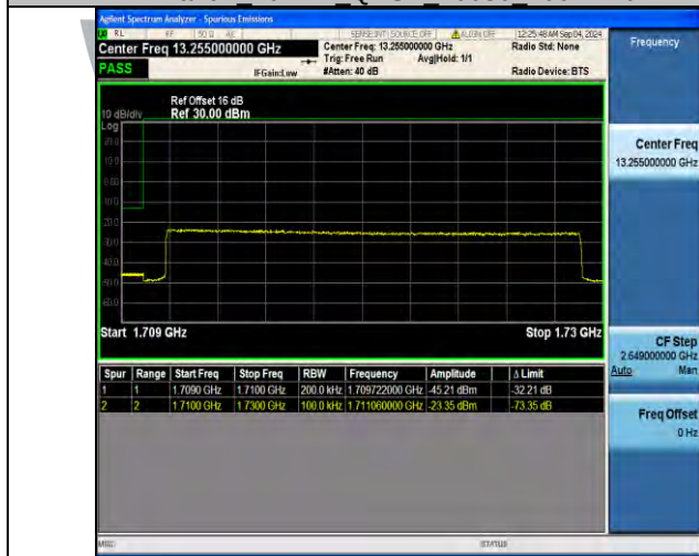
Band4 20MHz QPSK 20300 1RB#0
