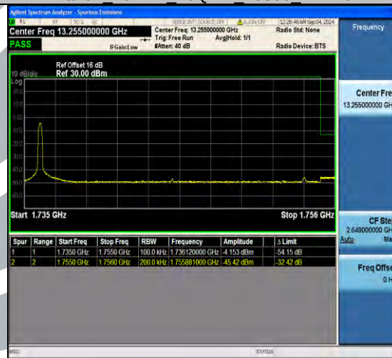
Band4 20MHz 16QAM 20300 100RB#0
