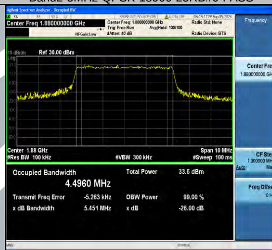
Band2-5MHz-QPSK-18800-25RB#0-PASS
