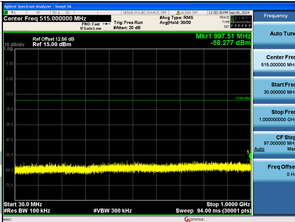
BLE_2M-Ant1-2404-30~1000-PASS
