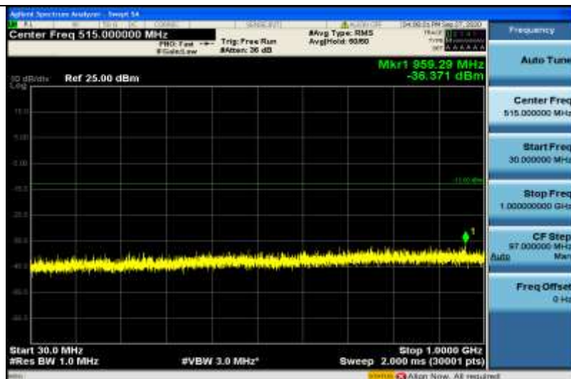
Band2-15MHz-16QAM-19125-1RB#0-Range2:1000~5000MHz
