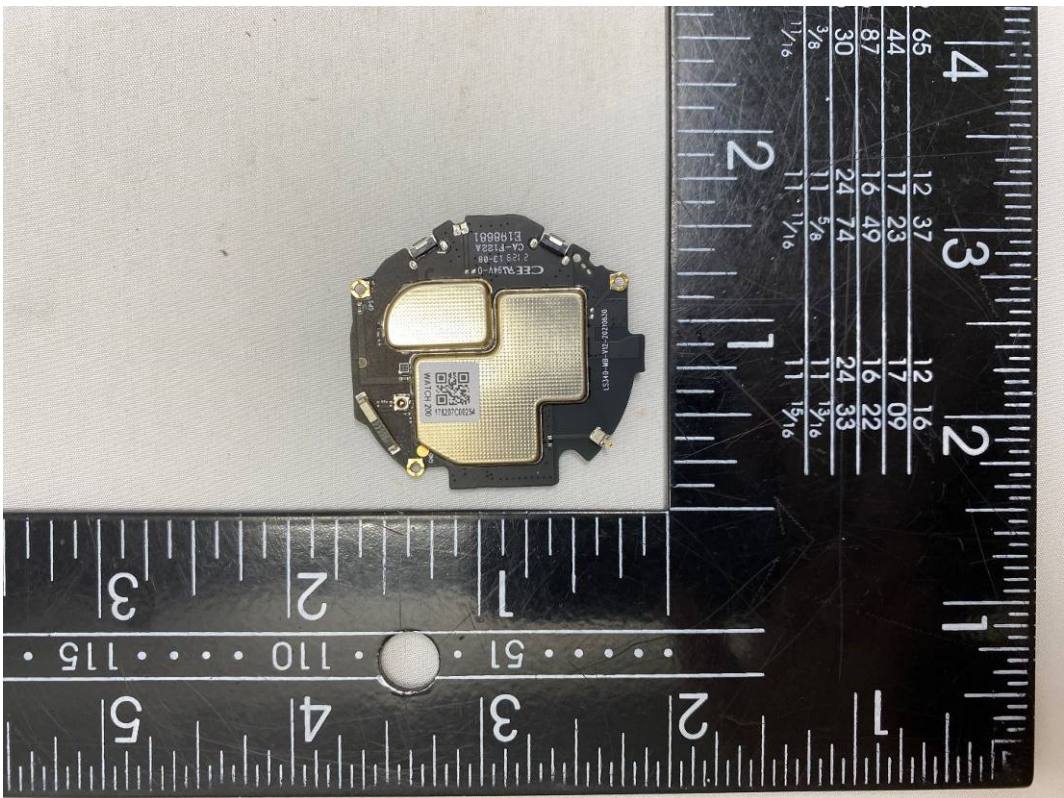
Fig. 5. PCB veiw-02
