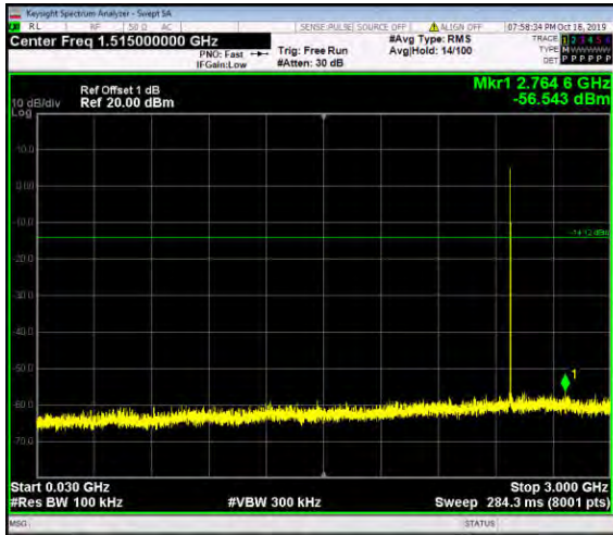
30MHz-3GHz
