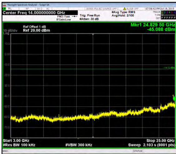
3GHz-25GHz
