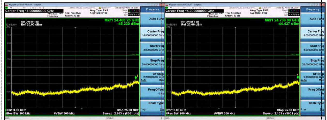
3GHz-25GHz
