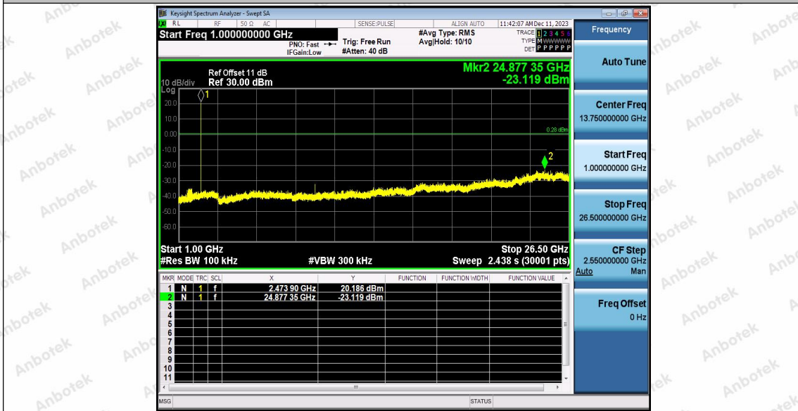
2.4G_Ant1_2474.1_1000~26500
