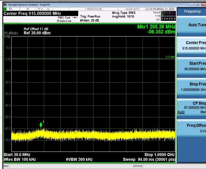
2.4G_Ant1_2439_30~1000
