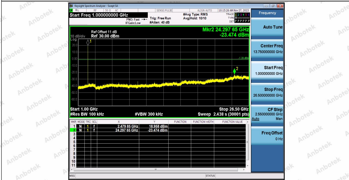
2.4G_Ant1_2479.8_1000~26500
