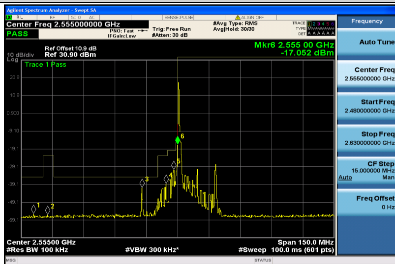
Band41-10MHz-QPSK-40290-1RB#0
