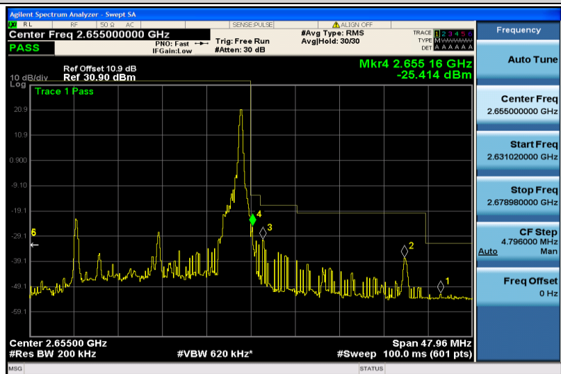
Band41-20MHz-QPSK-41140-1RB#99
