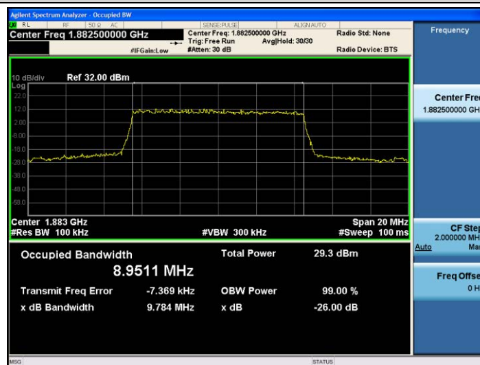
Band25-10MHz-QPSK-26365-50RB#0-8.9511
