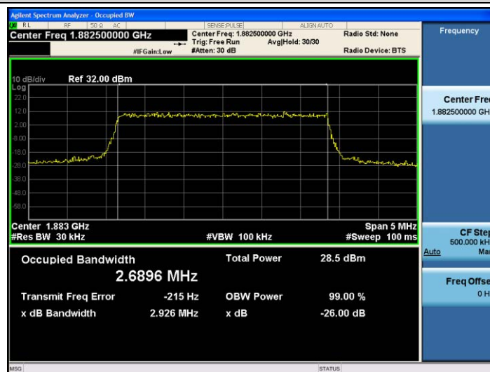
Band25-3MHz-QPSK-26365-15RB#0-2.6896
