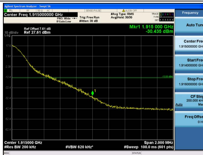
Band25-20MHz-16QAM-26590-1RB#99
