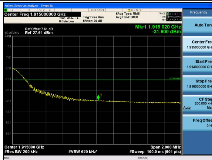
Band25-20MHz-QPSK-26590-100RB#0
