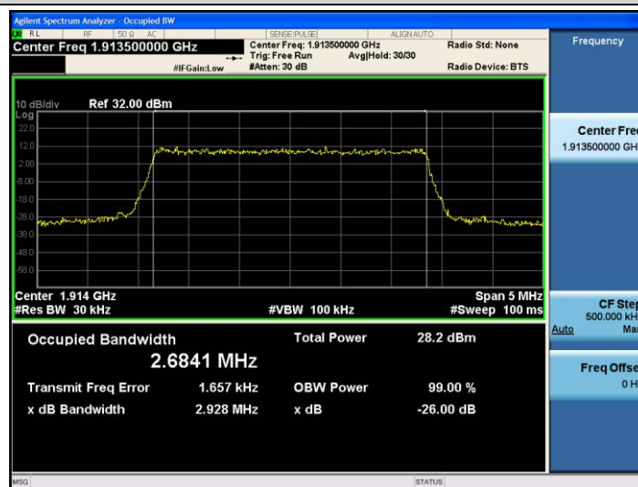
Band25-3MHz-QPSK-26675-15RB#0-2.6841
