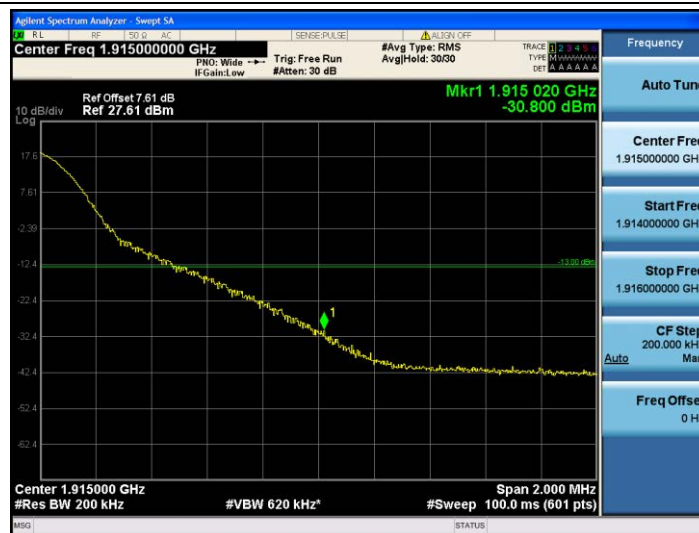
Band25-20MHz-QPSK-26590-1RB#99
