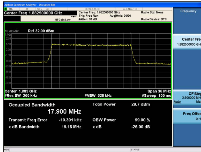
Band25-20MHz-QPSK-26365-100RB#0-17.900
