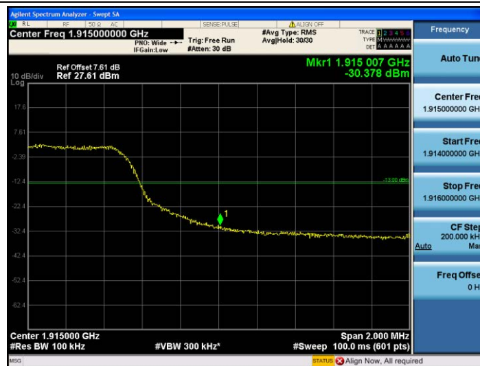
Band25-10MHz-QPSK-26640-50RB#0
