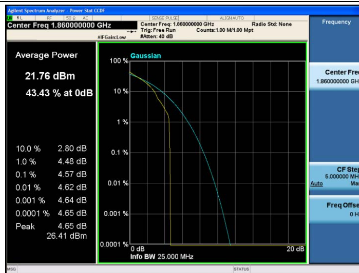
Band25-20MHz-QPSK-26140-1RB#0
