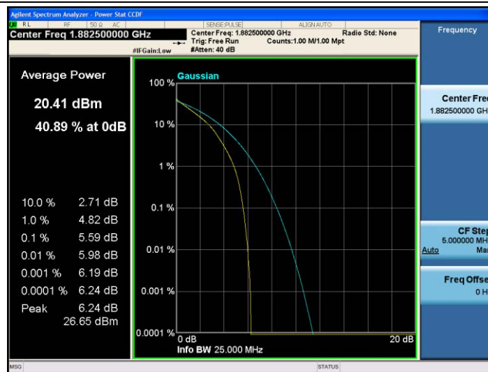
Band25-3MHz-QPSK-26365-15RB#0
