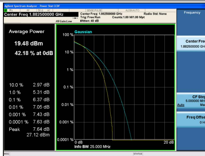
Band25-20MHz-16QAM-26365-100RB#0
