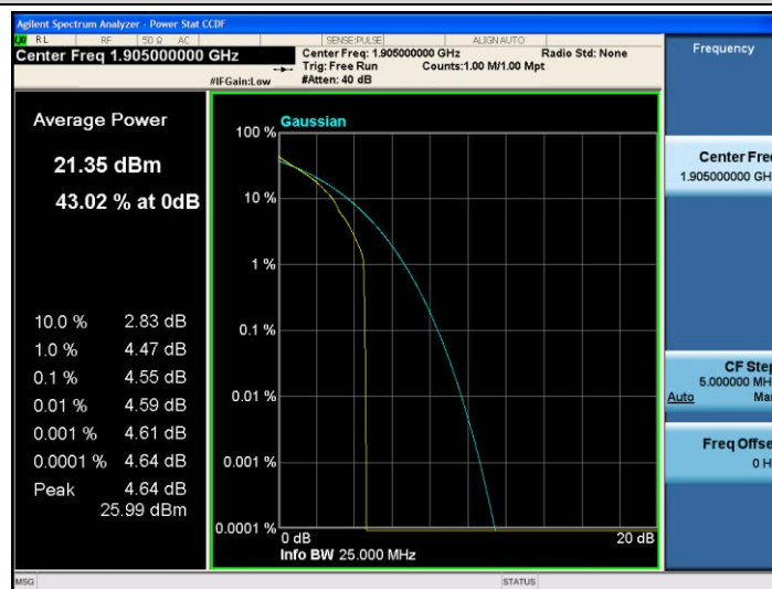
Band25-20MHz-QPSK-26590-1RB#0
