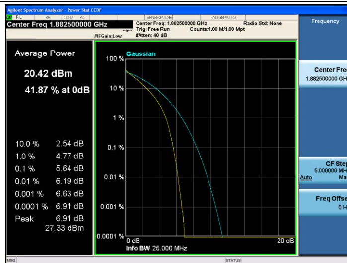
Band25-10MHz-QPSK-26365-50RB#0
