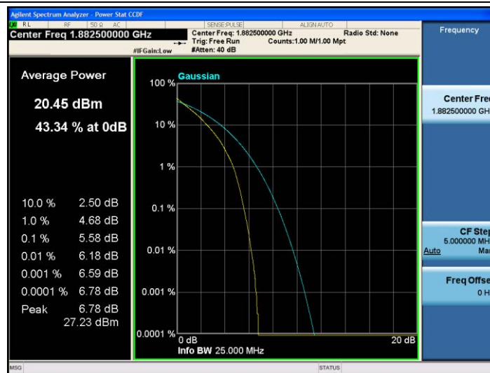
Band25-20MHz-QPSK-26365-100RB#0
