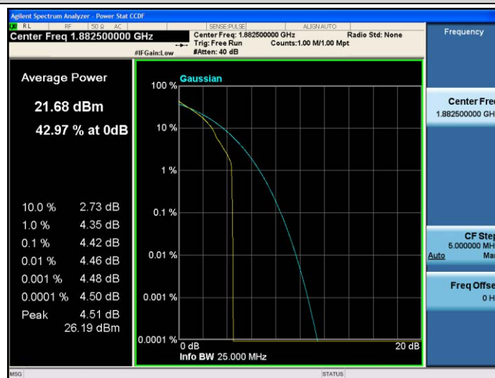
Band25-20MHz-QPSK-26365-1RB#0
