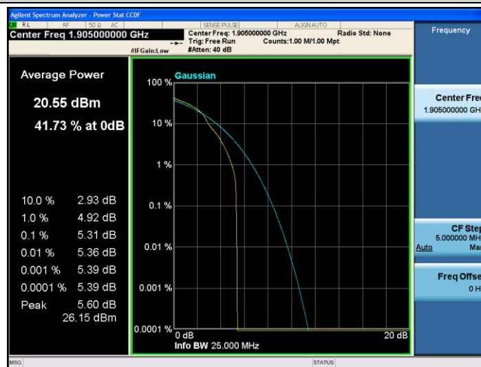
Band25-20MHz-16QAM-26590-1RB#0
