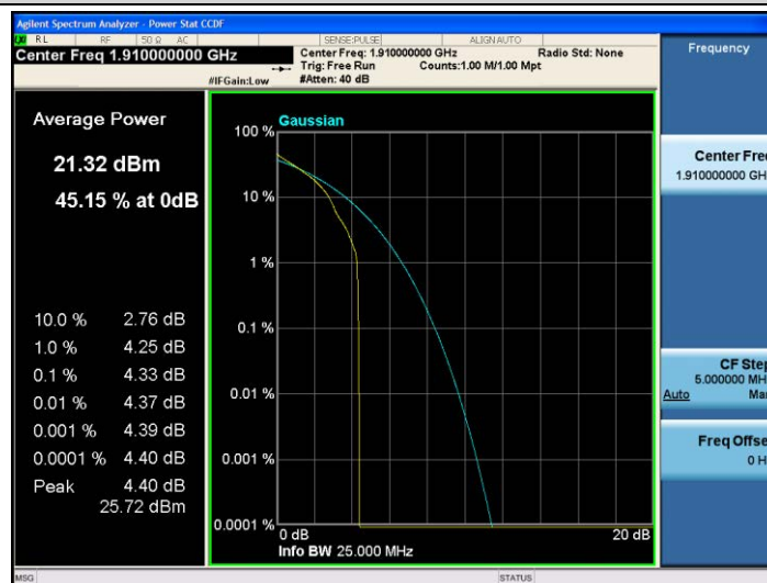
Band25-10MHz-QPSK-26640-1RB#0
