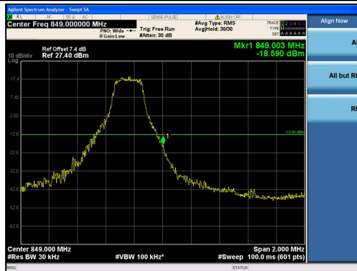
Band5-3MHz-QPSK-20635-1RB#14
