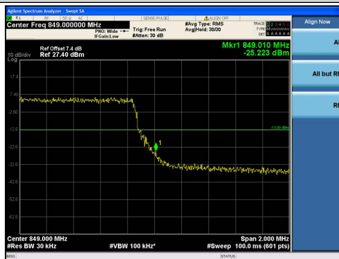
Band5-3MHz-QPSK-20635-15RB#0
