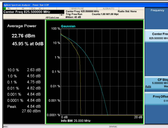
Band5-3MHz-QPSK-20415-1RB#0
