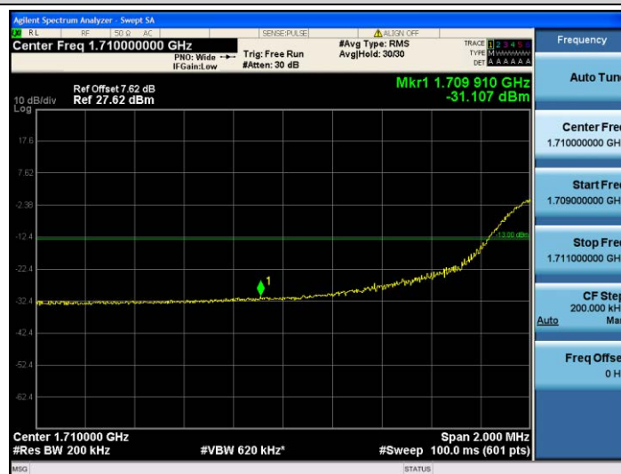
Band4-20MHz-QPSK-20050-100RB#0
