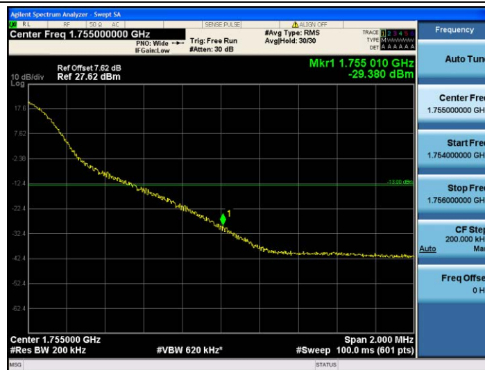
Band4-20MHz-QPSK-20300-1RB#99
