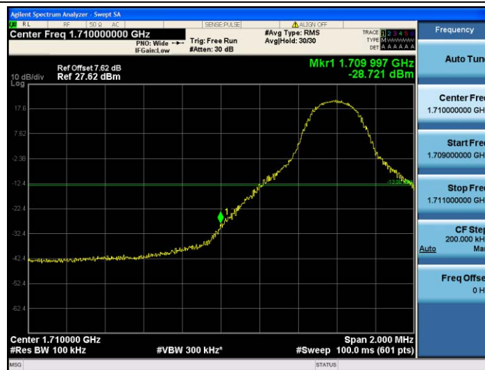
Band4-10MHz-QPSK-20000-1RB#0
