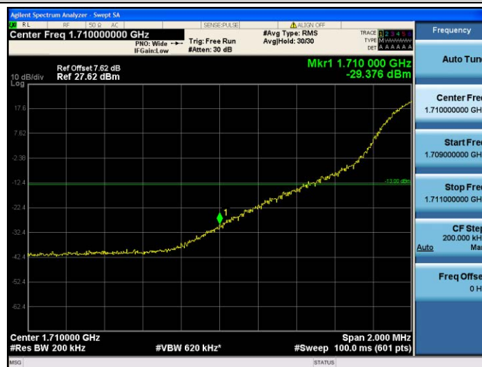
Band4-20MHz-QPSK-20050-1RB#0
