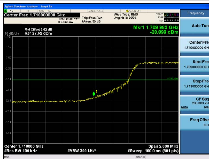
Band4-10MHz-QPSK-20000-50RB#0
