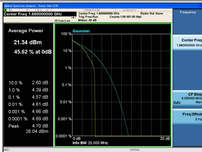
Band2-3MHz-QPSK-18900-1RB#0
