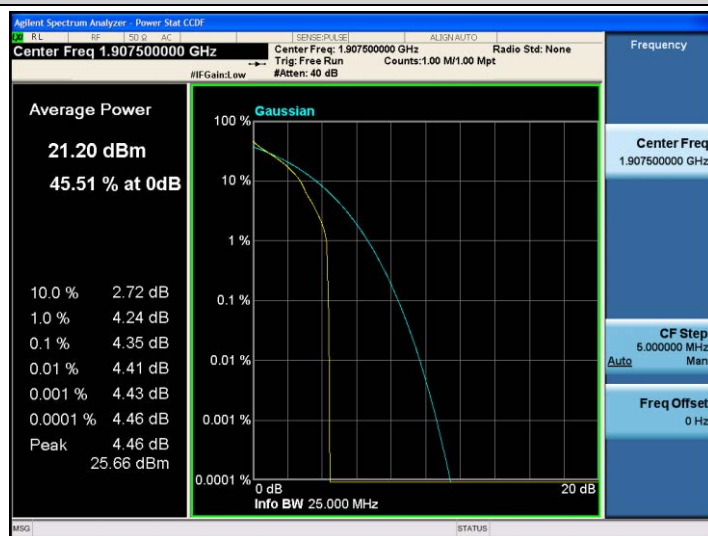
Band2-5MHz-QPSK-19175-1RB#0
