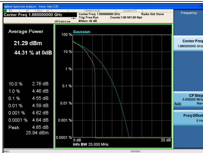
Band2-5MHz-QPSK-18900-1RB#0
