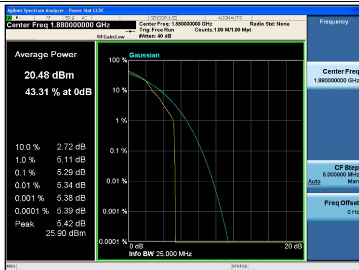
Band2-5MHz-16QAM-18900-1RB#0
