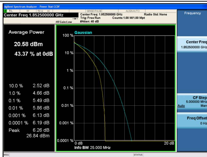
Band2-5MHz-QPSK-18625-25RB#0
