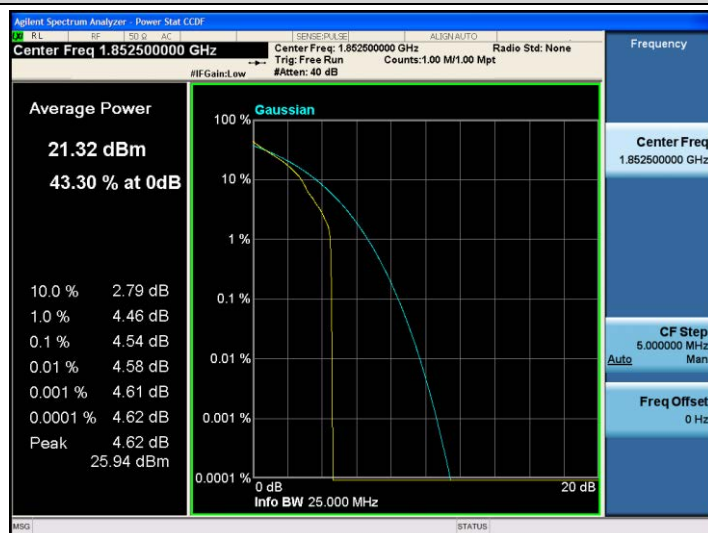
Band2-5MHz-QPSK-18625-1RB#0
