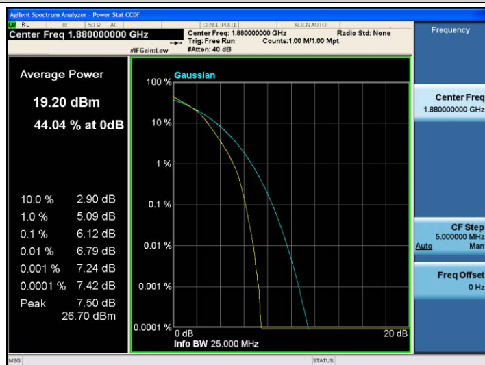
Band2-20MHz-16QAM-18900-100RB#0
