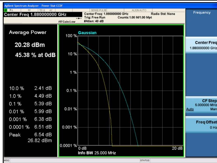
Band2-20MHz-QPSK-18900-100RB#0
