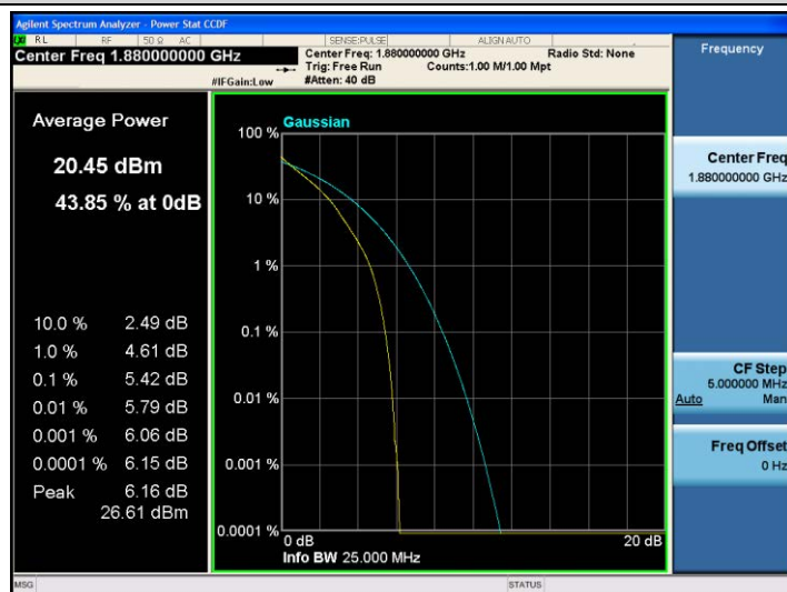
Band2-5MHz-QPSK-18900-25RB#0
