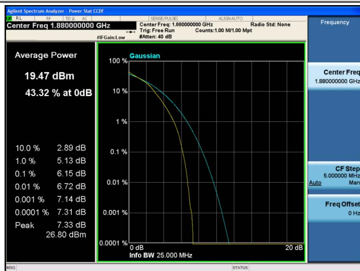
Band2-10MHz-16QAM-18900-50RB#0
