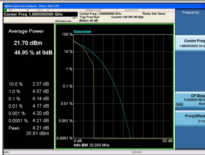
Band2-20MHz-QPSK-18900-1RB#0
