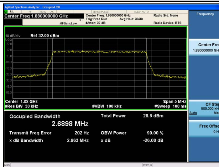
Band2-3MHz-QPSK-18900-15RB#0-2.6898
