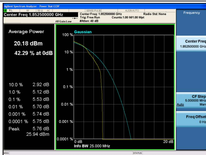
Band2-5MHz-16QAM-18625-1RB#0
