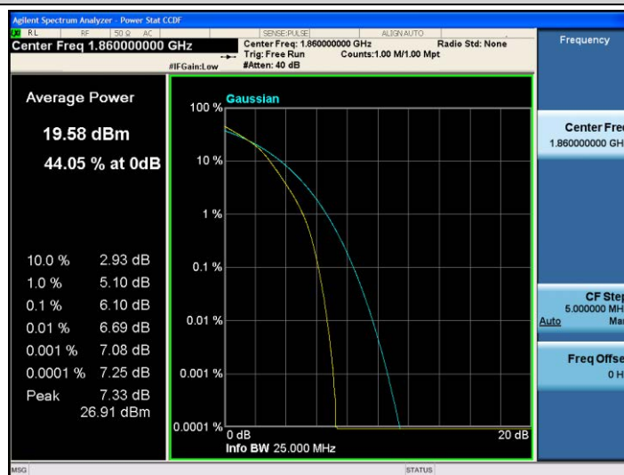
Band2-20MHz-16QAM-18700-100RB#0
