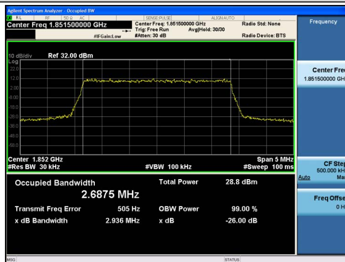
Band2-3MHz-QPSK-18615-15RB#0-2.6875
