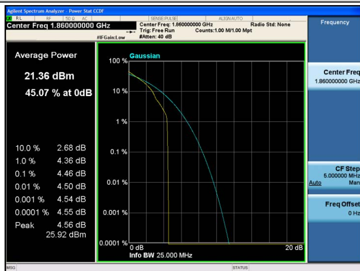
Band2-20MHz-QPSK-18700-1RB#0
