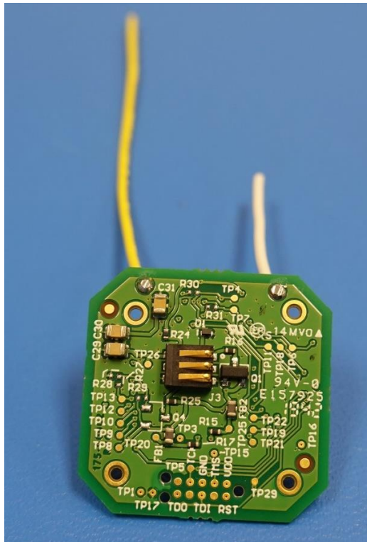
Relay PCBA bottom :
