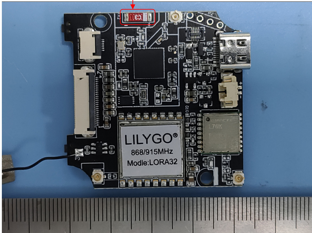
BLE Antenna
