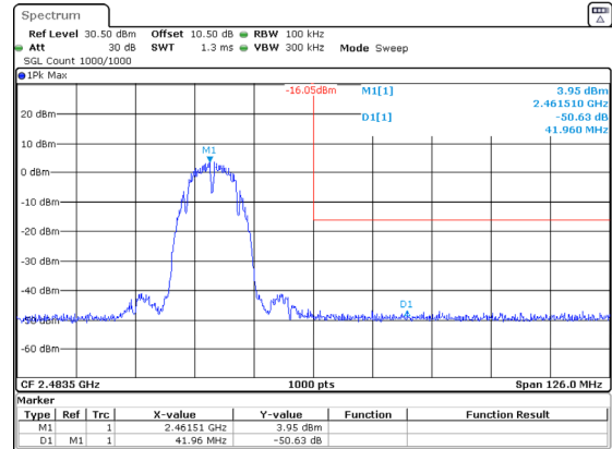
802.11b_2462MHz
