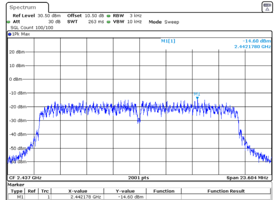
802.11n20_2437MHz
