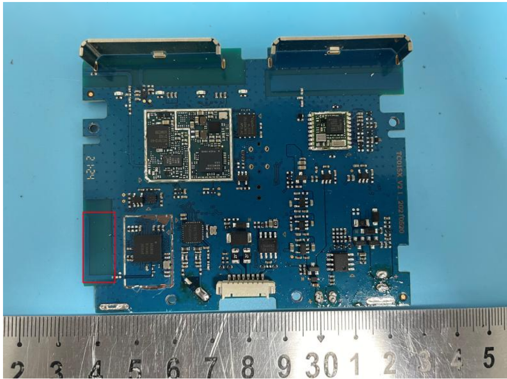
Antenna-NFC
