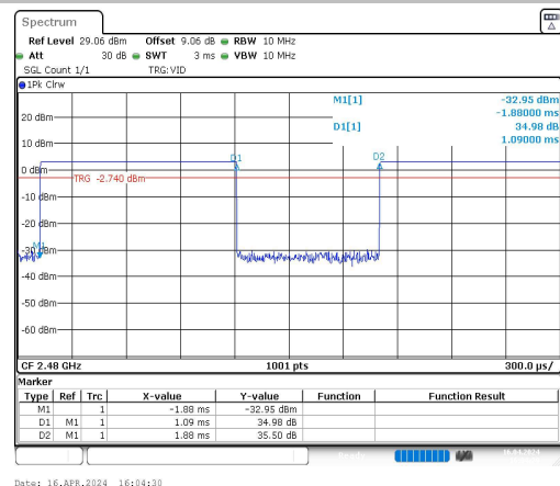
NTNV-BLE_2M-Ant1-2480
