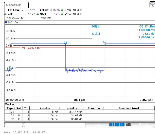
NTNV-BLE_2M-Ant1-2402
