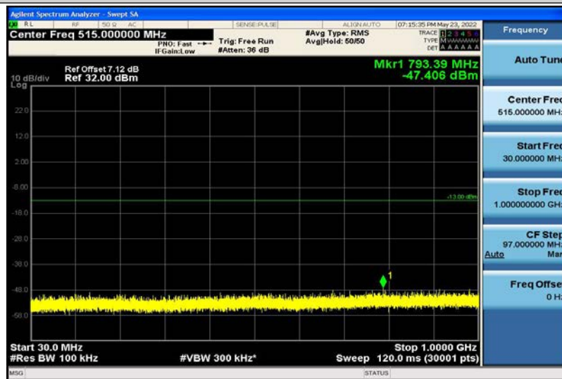
Band4-3MHz-QPSK-19965-1RB#0-30~1000MHz
