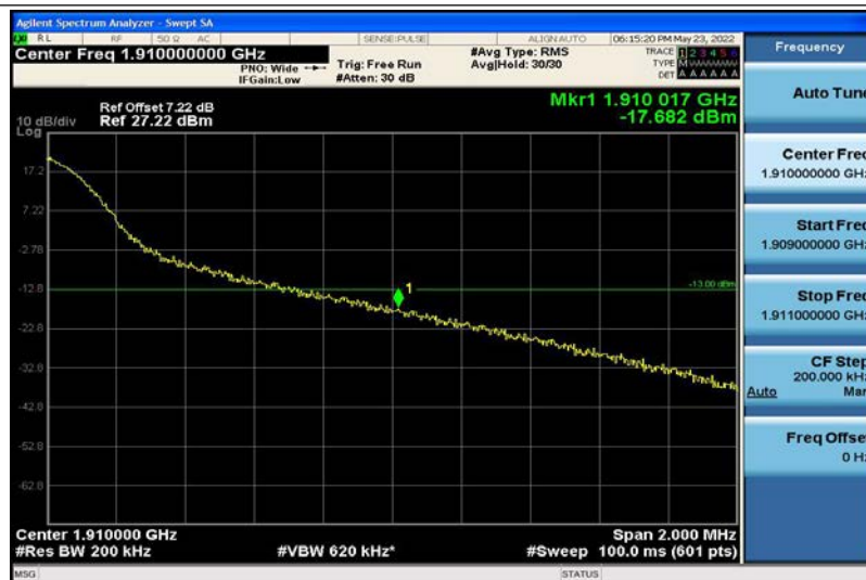
Band2-20MHz-QPSK-19100-1RB#99
