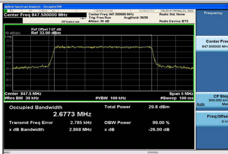
Band5-3MHz-QPSK-20635-15RB#0-2.6773
