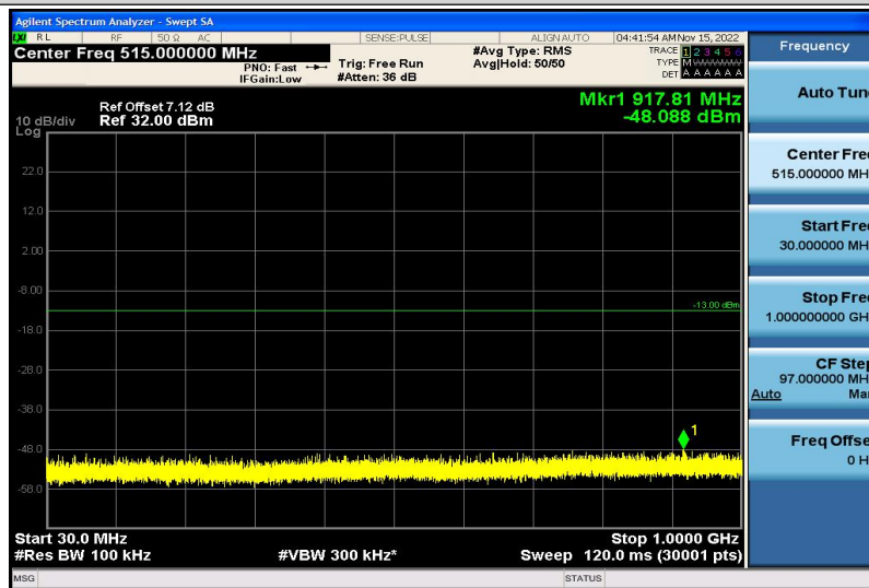
Band66-20MHz-QPSK-132572-1RB#0-30~1000MHz
