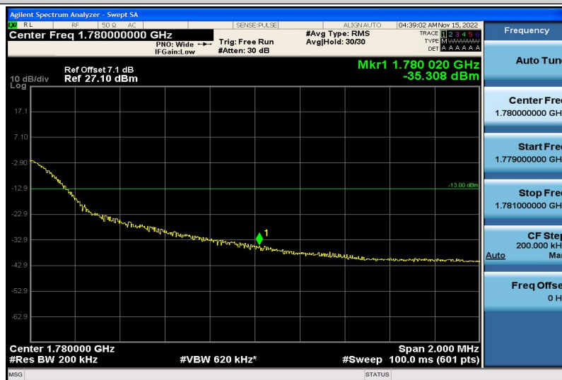
Band66-20MHz-QPSK-132572-100RB#0
