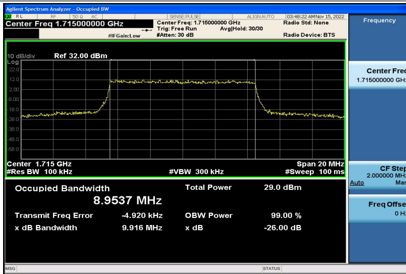
Band66-10MHz-QPSK-132022-50RB#0-8.9537
