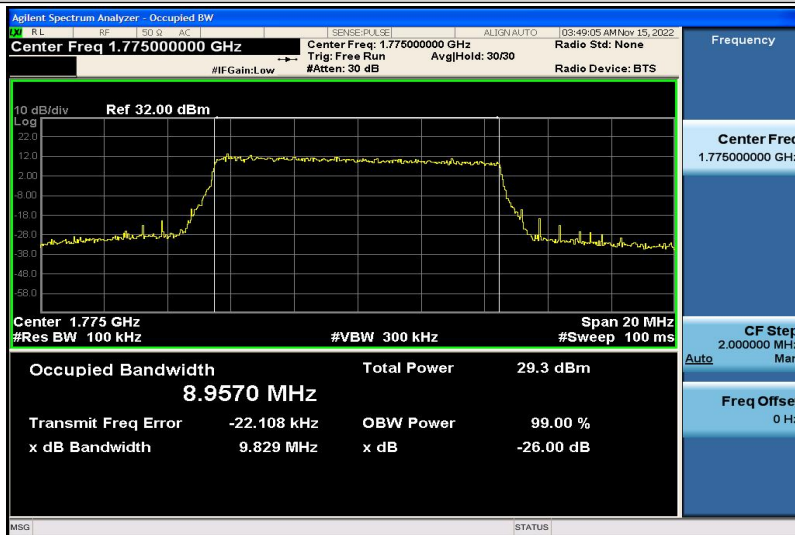
Band66-10MHz-QPSK-132622-50RB#0-8.9570
