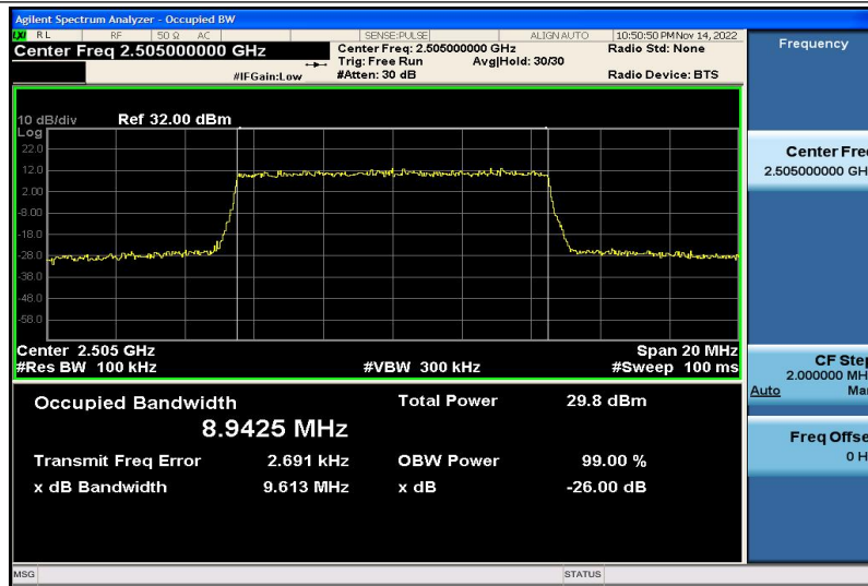
Band7-10MHz-QPSK-20800-50RB#0-8.9425
