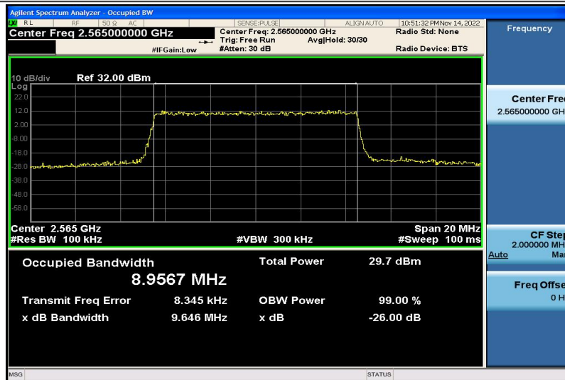
Band7-10MHz-QPSK-21400-50RB#0-8.9567
