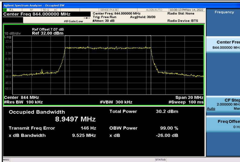
Band5-10MHz-QPSK-20600-50RB#0-8.9497
