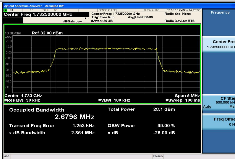
Band4-3MHz-QPSK-17325-15RB#0-2.6796
