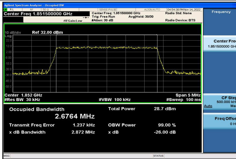
Band2-3MHz-QPSK-18615-15RB#0-2.6764
