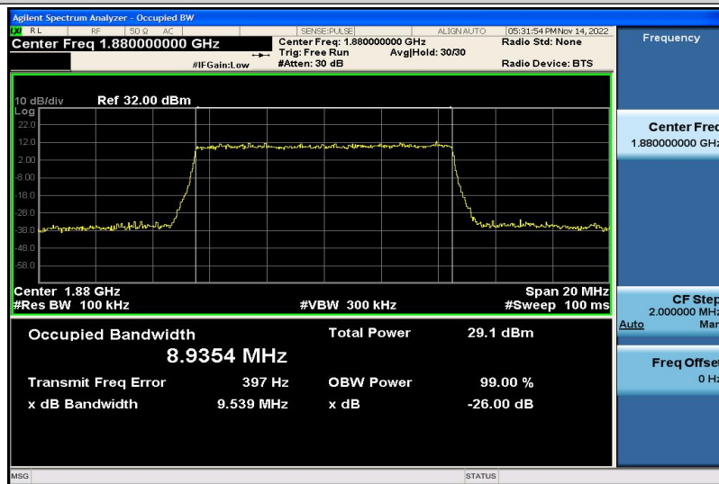
Band2-10MHz-QPSK-18900-50RB#0-8.9354
