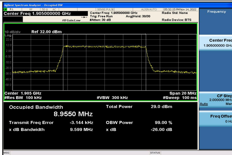
Band2-10MHz-QPSK-19150-50RB#0-8.9550
