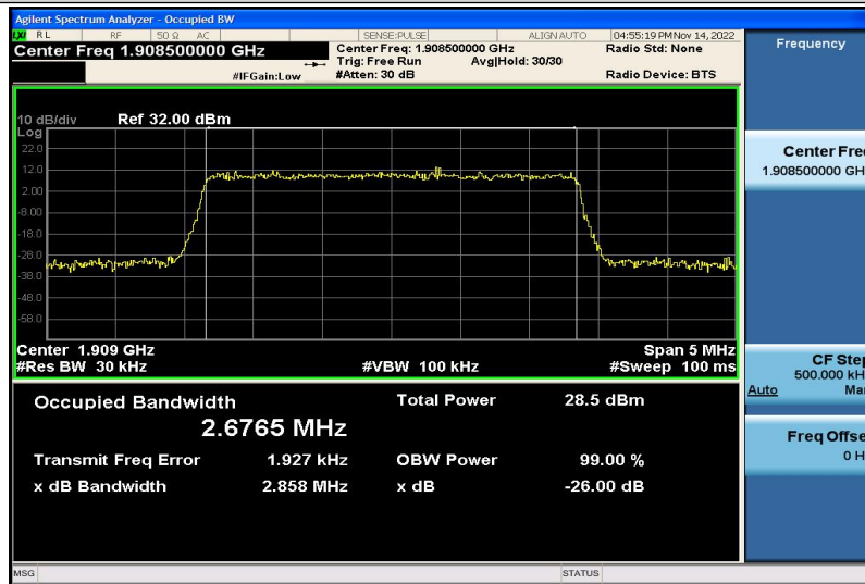
Band2-3MHz-QPSK-19185-15RB#0-2.6765
