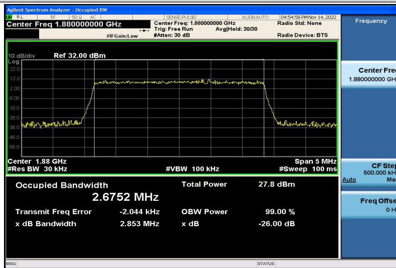
Band2-3MHz-QPSK-18900-15RB#0-2.6752
