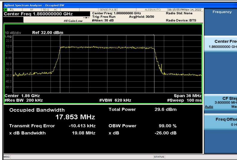
Band2-20MHz-QPSK-18700-100RB#0-17.853
