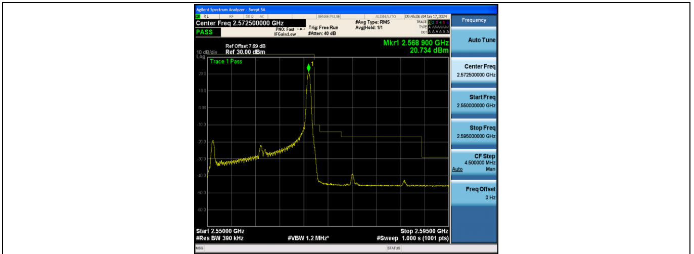
Band7_20MHz_QPSK_21350_1RB#99
