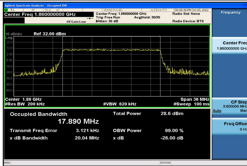
Band2-20MHz-QPSK-18700-100RB#0-17.890
