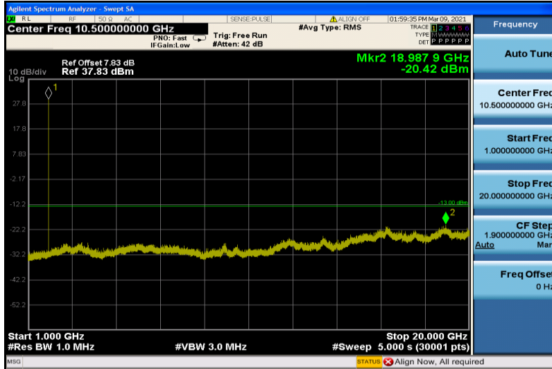
GSM1900-661-1000~20000
