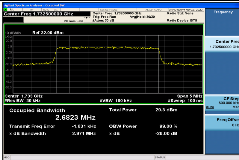
Band4-3MHz-QPSK-17325-15RB#0-2.6823
