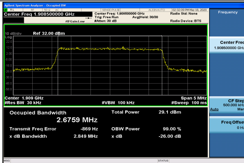
Band2-3MHz-QPSK-19185-15RB#0-2.6759
