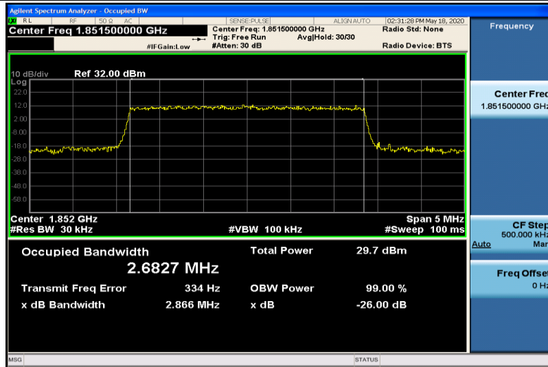
Band2-3MHz-QPSK-18615-15RB#0-2.6827
