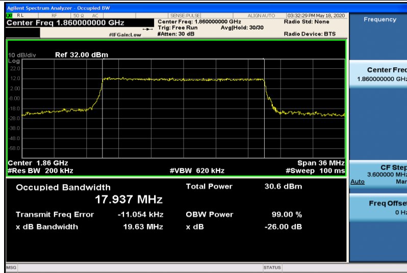
Band2-20MHz-QPSK-18700-100RB#0-17.937
