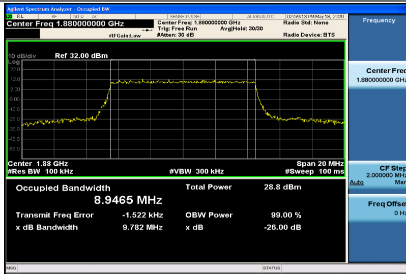
Band2-10MHz-16QAM-18900-50RB#0-8.9465
