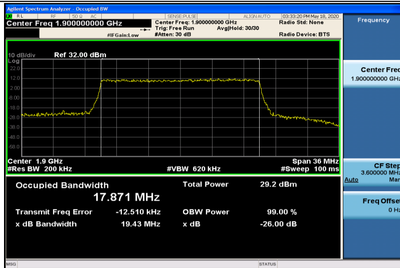
Band2-20MHz-16QAM-19100-100RB#0-17.871
