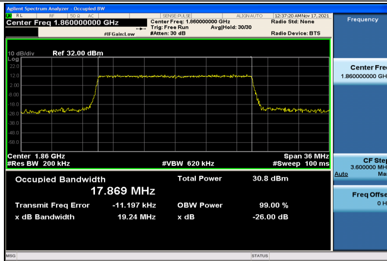
Band2-20MHz-QPSK-18700-100RB#0-17.869
