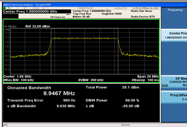
Band2-10MHz-16QAM-18900-50RB#0-8.9467
