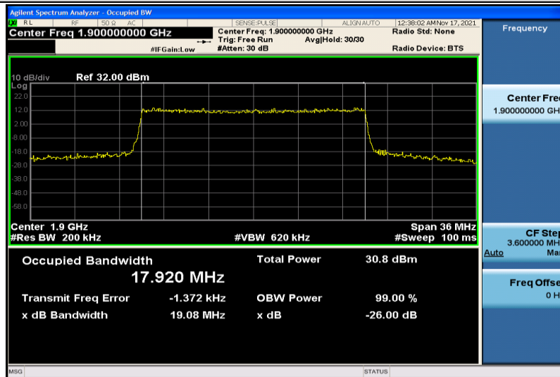
Band2-20MHz-QPSK-19100-100RB#0-17.920
