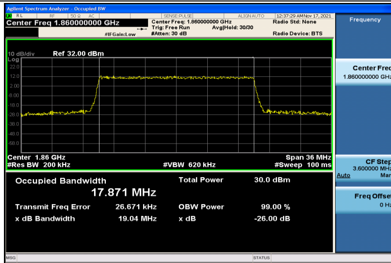
Band2-20MHz-16QAM-18700-100RB#0-17.871
