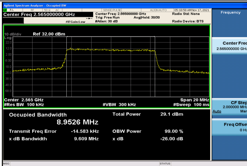
Band7-10MHz-QPSK-21400-50RB#0-8.9526
