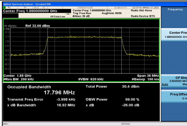
Band2-20MHz-QPSK-18900-100RB#0-17.796
