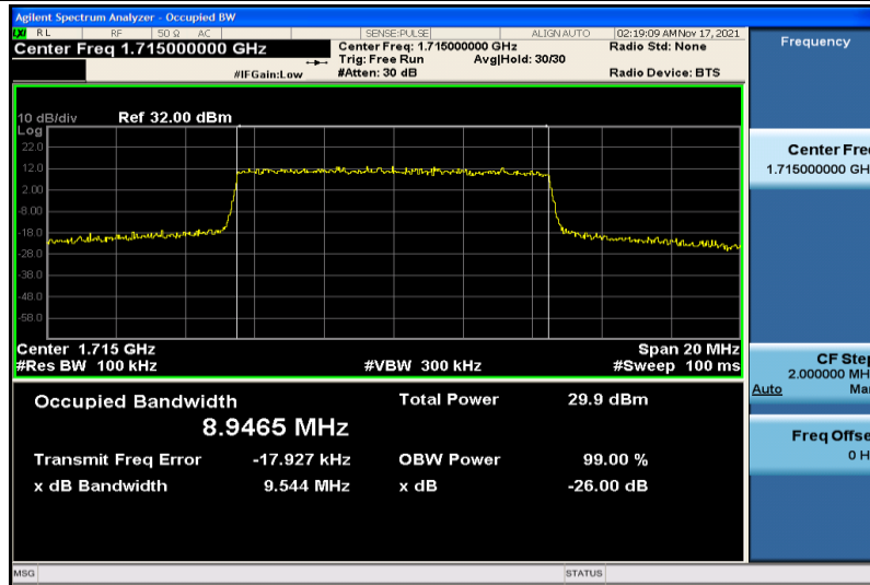
Band4-10MHz-QPSK-20000-50RB#0-8.9465
