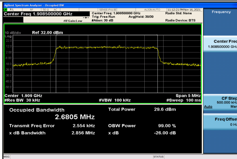
Band2-3MHz-QPSK-19185-15RB#0-2.6805
