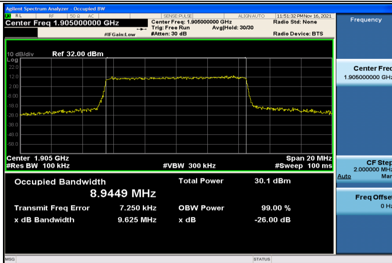
Band2-10MHz-QPSK-19150-50RB#0-8.9449
