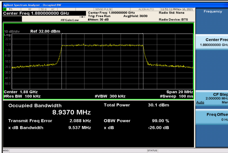
Band2-10MHz-QPSK-18900-50RB#0-8.9370
