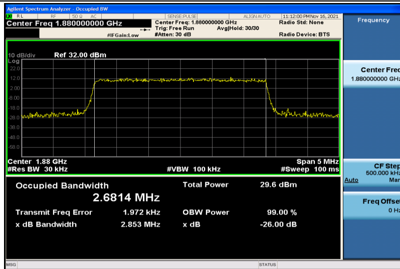
Band2-3MHz-QPSK-18900-15RB#0-2.6814
