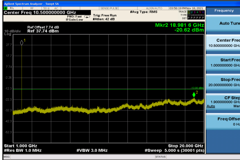
EGPRS1900-661-1000~20000
