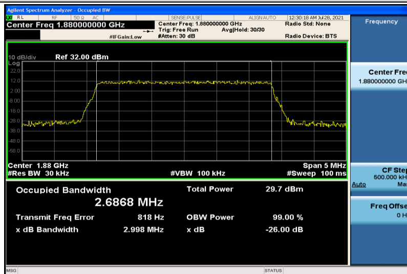
Band2-3MHz-QPSK-18900-15RB#0-2.6868
