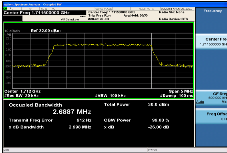
Band4-3MHz-QPSK-19965-15RB#0-2.6887
