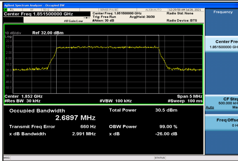
Band2-3MHz-QPSK-18615-15RB#0-2.6897
