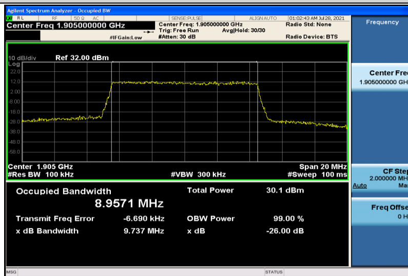
Band2-10MHz-QPSK-19150-50RB#0-8.9571
