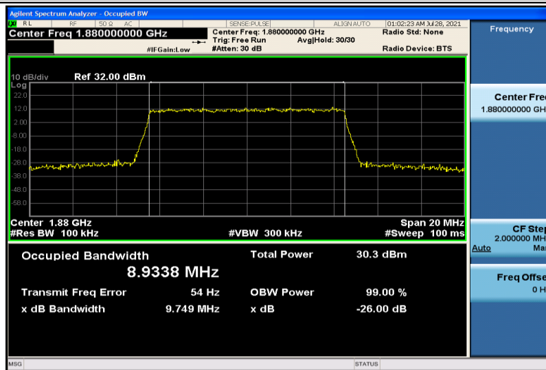
Band2-10MHz-QPSK-18900-50RB#0-8.9338
