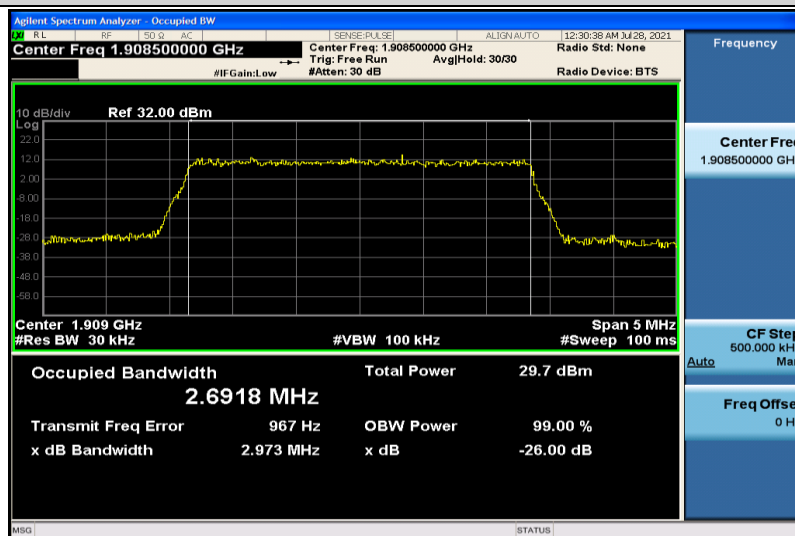
Band2-3MHz-QPSK-19185-15RB#0-2.6918
