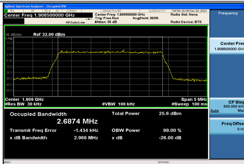
Band2-3MHz-QPSK-19185-15RB#0-2.6874
