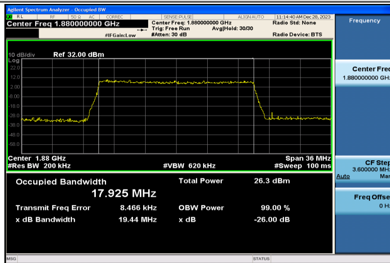
Band2-20MHz-QPSK-18900-100RB#0-17.925
