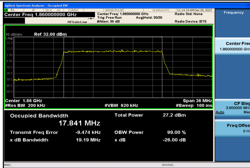
Band2-20MHz-QPSK-18700-100RB#0-17.841
