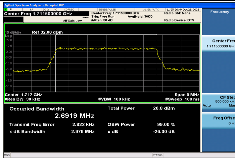
Band4-3MHz-QPSK-19965-15RB#0-2.6919
