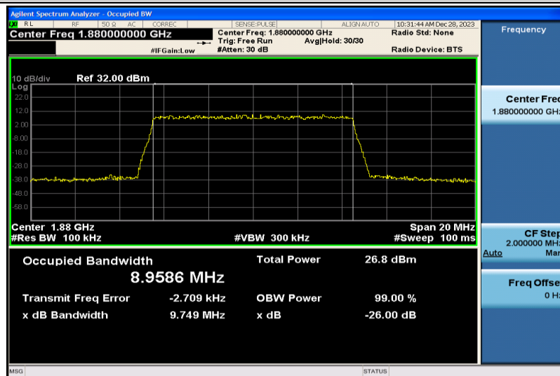
Band2-10MHz-QPSK-18900-50RB#0-8.9586
