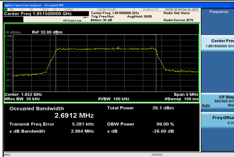
Band2-3MHz-QPSK-18615-15RB#0-2.6912
